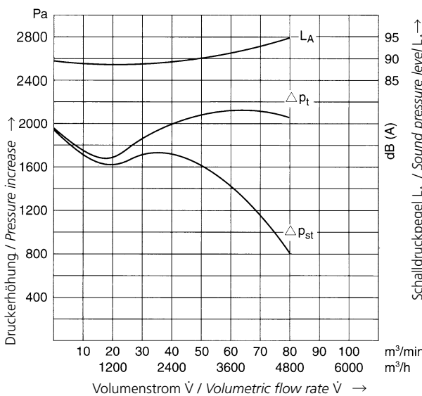
50 Hz
