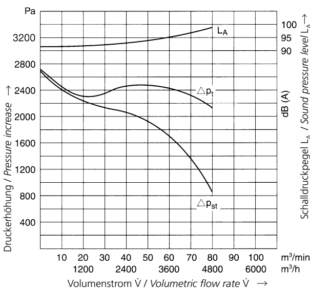
60 Hz
