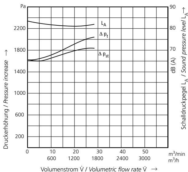
60 Hz
