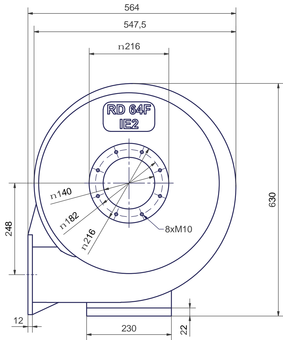
Ansicht A
